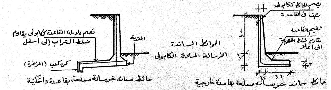
شكل رقم (36) الأشكال المختلفة من الحوائط الساندة
