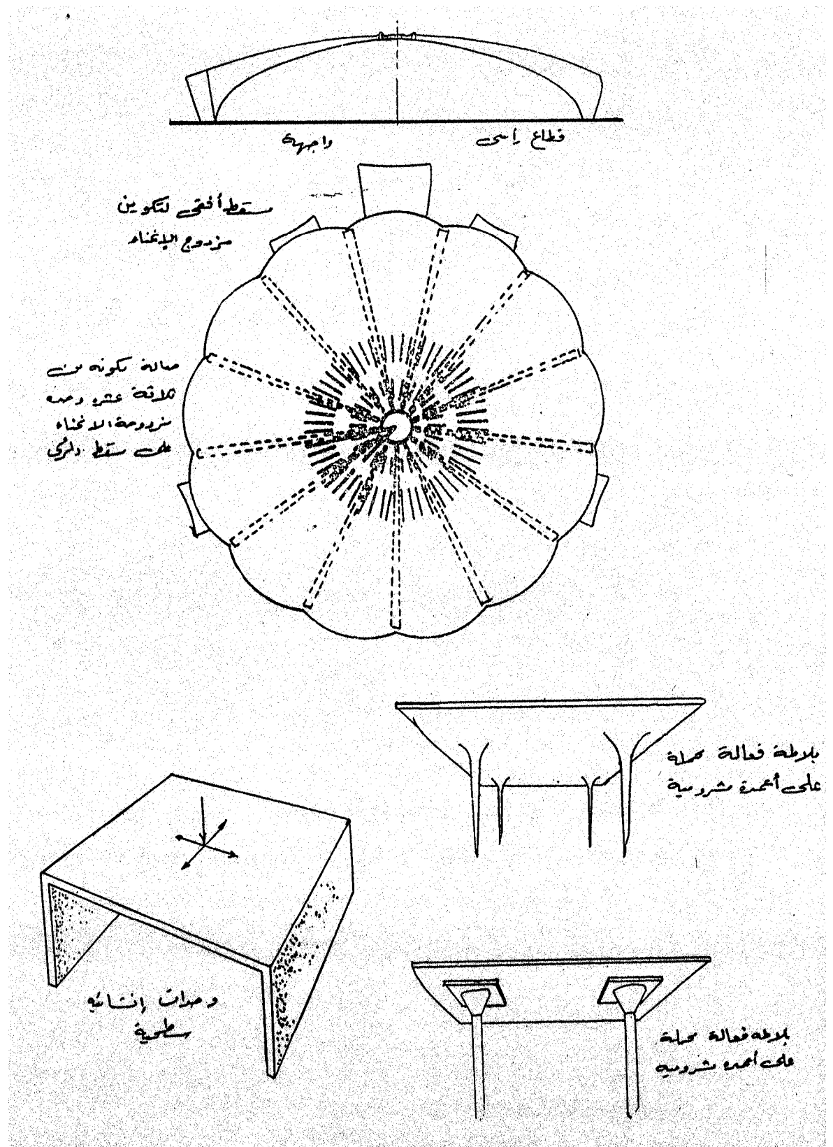
شكل رقم (43) التكوينات بالسطح الإنشائية الفعالة
