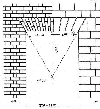
عقد مستقيم
