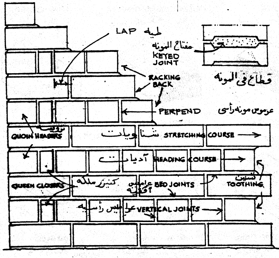
شكل (29): واجهة لمباني حائط وعليها المصطلحات العامة لرص الطوب.
