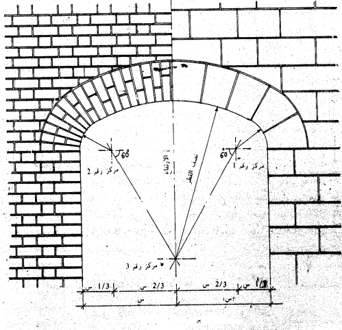
عقد مخموس
