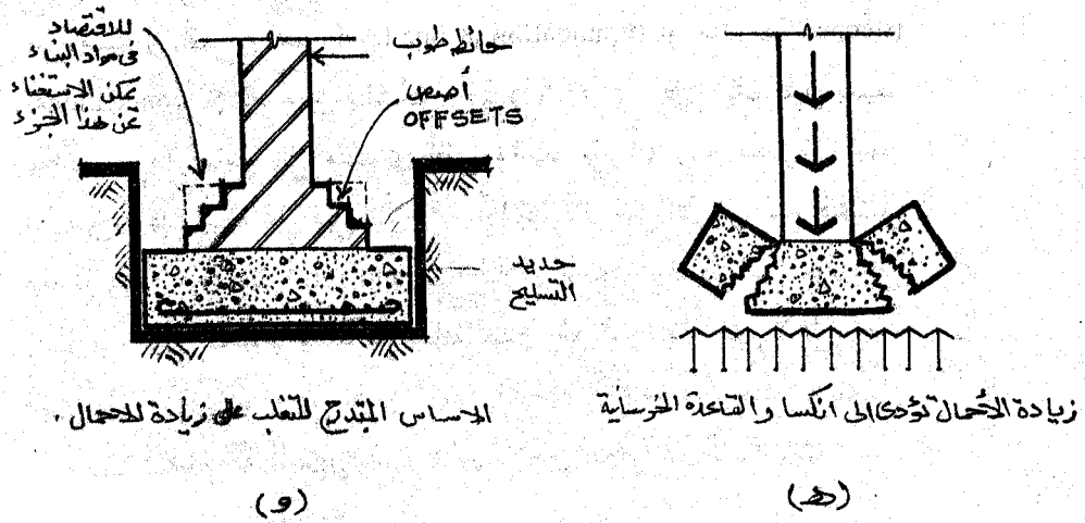
شكل رقم (16): مبادئ تصميم أساسات القواعد السطحية للمباني الحوائط الحاملة.
