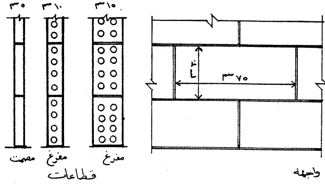
بلوكات جبسية
