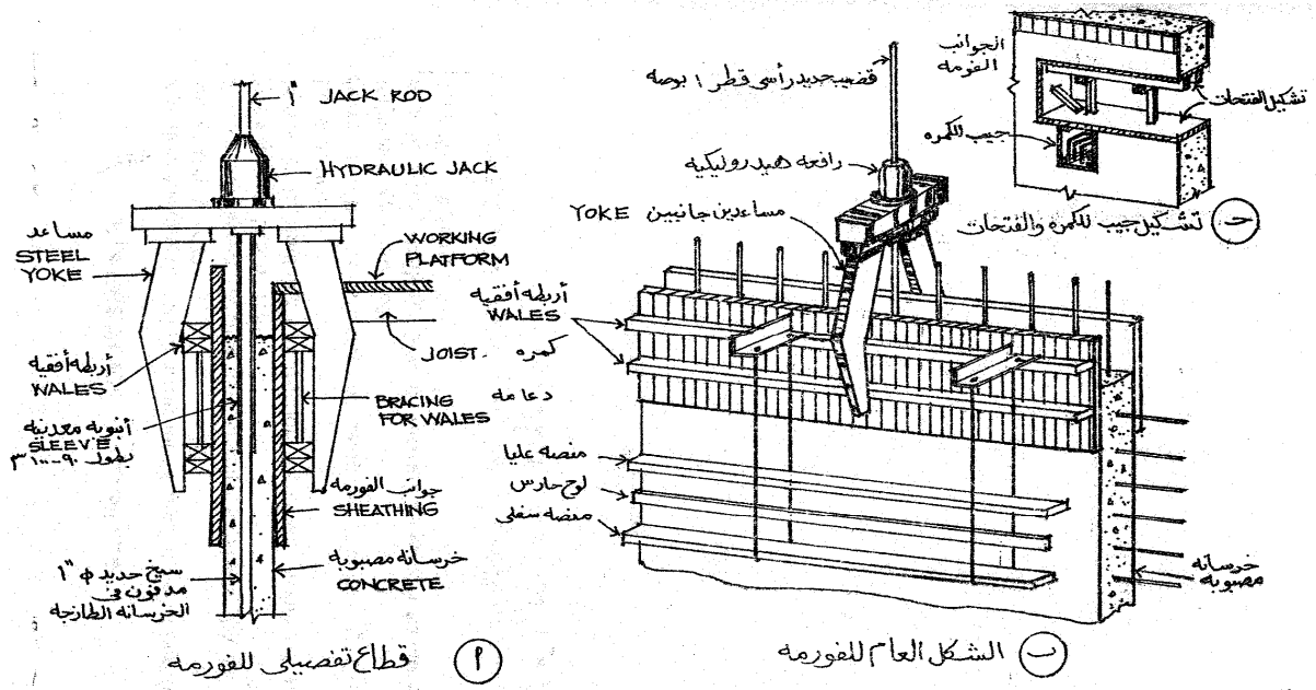
شكل (8): طريقة الشدات المنزلاقة.
