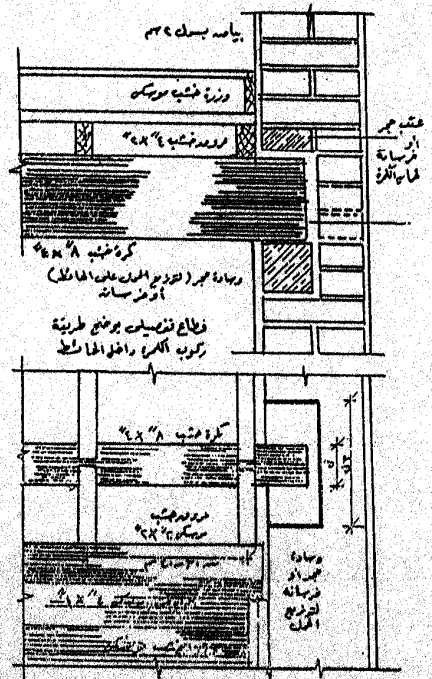
شکل رقم (45) مسقط أفقي وقطاعات تفصيلية لسقف خشب مزدوج
