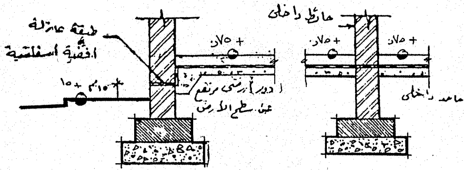
قطاع رأسي يوضح الطبقة العازلة لجوهر الأرض مرتفع عن سطح الأرض قطاع رأسي في حائط داخلي يوضح استمرار عازل الرطوبة
