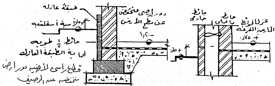
استخدام الحوائط المرفقة للضوء الحراري
