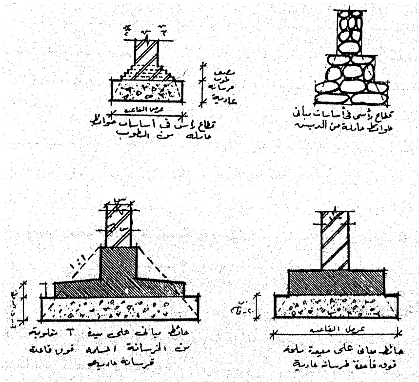
شکل رقم (17): الأنواع المختلفة للأساسات السطحية للمباني الحوائط الحاملة.
