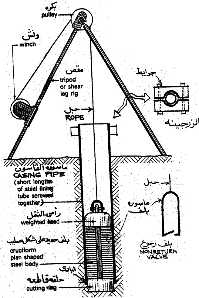
شكل رقم (12): ماكينة الجسات اليدوية (القايسون)
